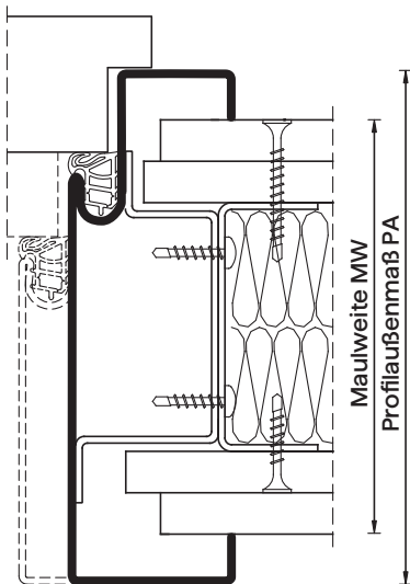
Normfalz/Doppelfalz
